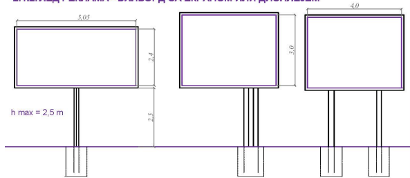
Прилог 2. Изглед билборда са екраном или дисплејем
