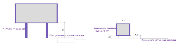
Прилог 10. Услови постављања огласних паноа поред бициклистичких стаза
