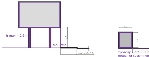
Прилог 9. Услови постављања огласних паноа поред и на пешачким стазама
