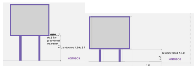
Прилог 12. Услови постављања огласних паноа поред коловоза
