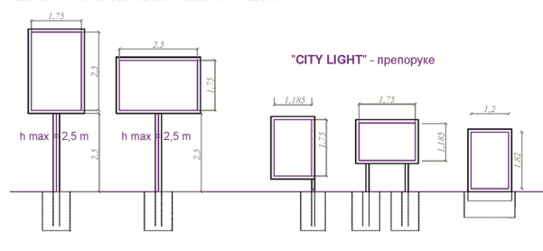
Прилог 4. Изглед огласног паноа типа "City Light"
